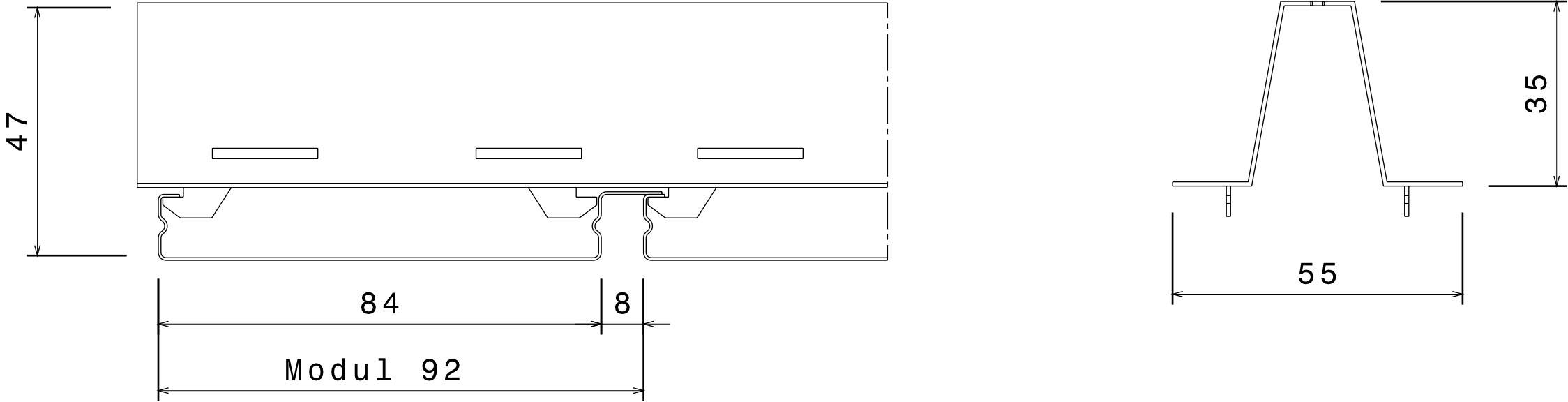
Trageschiene Typ HZF
