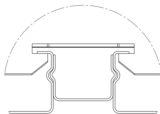
Detail A Füllprofil (FP)
