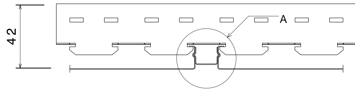
Trageschiene Typ VZF
